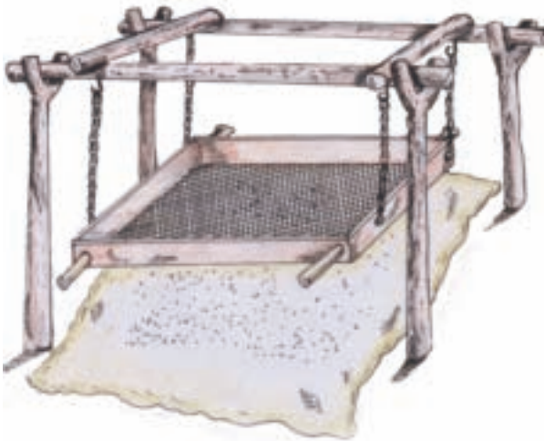
Modèle simple pour tamiser les semences de sorgho : grillage pour tamiser le sable avec un support.
